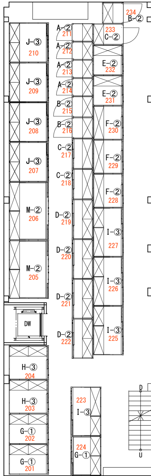
2階平面図 【34室】
