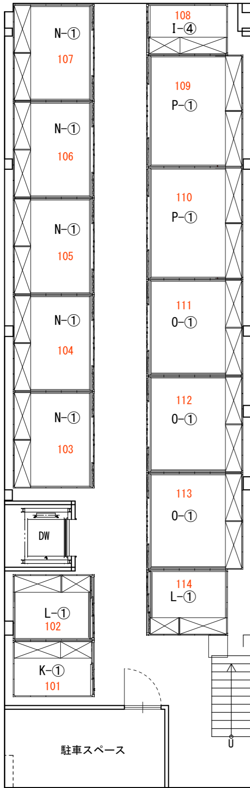
1階平面図 【14室】
